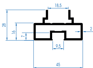
B Sección Perfil B
