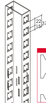
COLUMNA TROQUELADA 2 CARAS COLONNE PERFORATION SIMPLE 2 CÔTÉS UPRIGHT SINGLE SLOT CHANNEL 2 SIDES PIANTANA PERFORAZIONE SINGOLA 2 LATI 4815/13B 1337 mm
