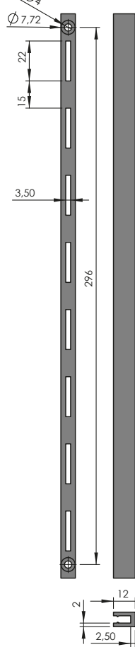
KADÍ EMPOTRABLE ALUMINIO
