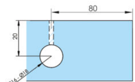
Muesca en OSLO de vidrio para cojinete 4921/022.
