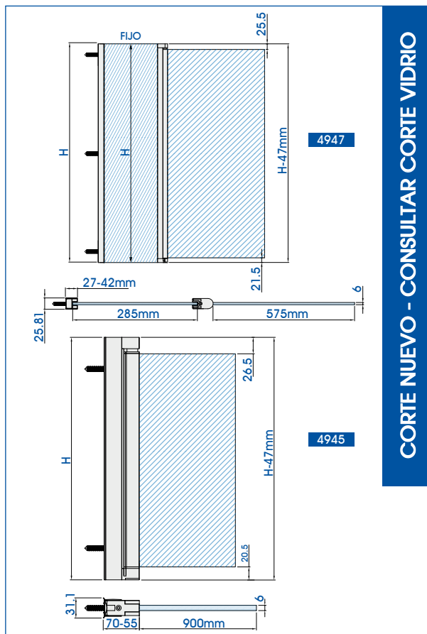
Medidas corte vidrio ROMA
