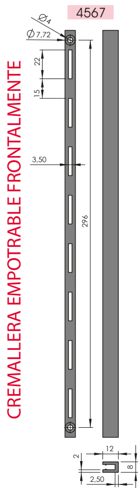
KADÍ EMPOTRABLE ALUMINIO
