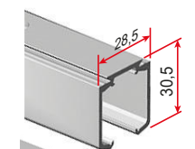
CARRIL SUPERIOR RAIL EN ALUMINIUM ALUMINIUM RAIL BINARIO IN ALLUMINIO *3480/101 FACTURACIÓN EN 2M., 3M Y 4M.
