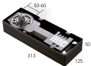
FRENO FERME-PORTE DOOR CLOSER CHIUDIORTA
