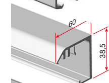
PERFIL DE ANCLAJE A PARED PROFIL D'ANCRAGE MURAL WALL ANCHOR PROFILE PROFILE PER FISSAGGIO A PARETE *3482/101 FACTURACIÓN EN 2M., 3M Y 4M.
