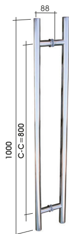
MANILLA DOBLE 100 CM POIGNEÉ DOUBLE 100 CM DOUBLE DOOR HANDLE 100 CM MANIGLIA DOPPIA 100 CM 1592/0..
