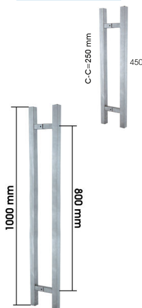
MANILLA DOBLE 45 CM POIGNEÉ DOUBLE 45 CM DOUBLE DOOR HANDLE 45 CM MANIGLIA DOPPIA 45 CM 1597/0..
