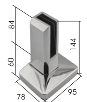
SOPORTE VIDRIO 90° ESQUINERO support de verre d'angle 90° 90° corner glass support supporto vetro angolare a 90°
