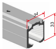
CARRIL SUPERIOR RAIL EN ALUMINIUM ALUMINIUM RAIL BINARIO IN ALUMINIO *3470/101 FACTURACIÓN EN 2M., 3M Y 4M.
