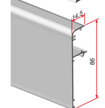
TAPA DE CARRIL SUPERIOR COUVERTURE DE RAIL SUPÉRIEUR TOP RAIL COVER COPERTURA SUPERIORE DEL BINARIO *3481/101 FACTURACIÓN EN 2M., 3M Y 4M.
