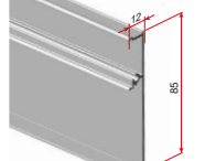
TAPA DE CARRIL SUPERIOR COUVERTURE DE RAIL SUPÉRIEURE TOP RAIL COVER COPERTURA SUPERIORE DEL BINARIO *3471/101 FACTURACIÓN EN 2M., 3M Y 4M.
