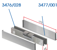
KIT DE 2 TAPAS PARA PINZAS. LOT DE 2 COUVERCLES POUR PINCES. SET OF 2 CAPS FOR CLAMP KIT 2 VELLETTA PINZA. *3477/001 Solo para KIT 3476
