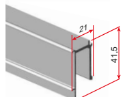
PERFIL PARA VIDRIO FIJO PROFIL POUR VERRE FIXE PROFILE FOR FIXED GLASS PROFLO PER VETRO FISSO *3475/101 FACTURACIÓN EN 2M., 3M Y 4M.
