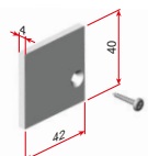
TAPA LATERAL DE CARRIL SUPERIOR COUVERTURE LATÉRALE DU RAIL SUPÉRIEUR TOP RAIL SIDE COVER COPERTURA LATERALE SUPERIORE *3473/001 Set dcha. izda.
