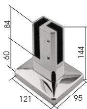
SOPORTE VIDRIO 90° ESQUINERO support de verre d'angle 90° 90° corner glass support supporto vetro angolare a 90°
