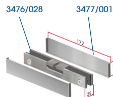
KIT DE 2 TAPAS PARA PINZAS LOT DE 2 COUVERCLES POUR PINCES SET OF 2 CAPS FOR CLAMP KIT 2 VELLETTA PINZA *3477/001 Solo para KIT 3476
