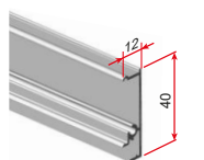
TAPA DE CARRIL SUPERIOR COUVERTURE DE RAIL SUPÉRIEURE TOP RAIL COVER COPERTURA SUPERIORE DEL BINARIO *3472/101 FACTURACIÓN EN 2M., 3M Y 4M.
