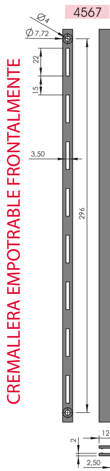
KADÍ EMPOTRABLE ALUMINIO
