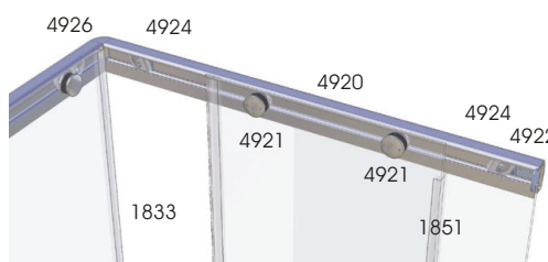
Ejemplo desglose kit 4029
