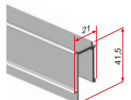
PERFIL PARA VIDRIO FIJO PROFIL POUR VERRE FIXE PROFILE FOR FIXED GLASS PROFLO PER VETRO FISSO *3475/101 FACTURACIÓN EN 2M., 3M Y 4M.
