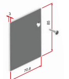
TAPA LATERAL DE CARRIL SUPERIOR COUVERTURE LATÉRALE DU RAIL SUPÉRIEUR TOP RAIL SIDE COVER COPERTURA LATERALE SUPERIORE *3474/001 Set dcha. izda.
