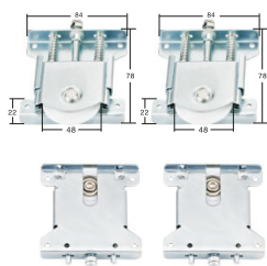
CARRIL INFERIOR DOBLE RAIL DOBLE INFERIEUR LOWER DOUBLE RAIL BINARIO DOPPIO INF. *1724/1..
