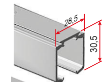
CARRIL SUPERIOR RAIL EN ALUMINIUM ALUMINIUM RAIL BINARIO IN ALUMINIO *3480/101 FACTURACIÓN EN 2M., 3M Y 4M.
