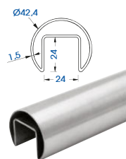
PROFILO PASAMANO Ø42.2 PROFIL GARDE-CORPS BALUSTRADE PROFIL PROFILO BALAUSTRAS INOX 316L *5100/122 Ø 42,4 mm
