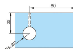
Muesca en OSLO de vidrio para cojinete 4921/022.
