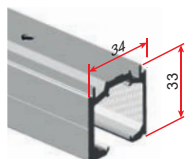
CARRIL SUPERIOR RAIL EN ALUMINIUM ALUMINIUM RAIL BINARIO IN ALLUMINIO *3470/101 FACTURACIÓN EN 2M, 3M Y 4M.
