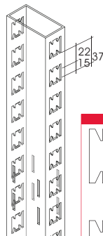
COLUMNA TROQUELADA 2 CARAS COLONNE PERFORATION SIMPLE 2 CÔTÉS UPRIGHT SINGLE SLOT CHANNEL 2 SIDES PIANTANA PERFORAZIONE SINGOLA 2 LATI 4815/13B 1337 mm
