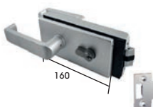
CERRADURA CON MANEJA SERRURE AVEC POIGNÉE DOOR LOCK WITH HANDLE SERRATURA CON MANIGLIA 5577/001 5577/00N
