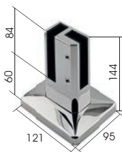
SOPORTE VIDRIO 90° ESQUINERO support de verre d'angle 90° 90° corner glass support supporto vetro angolare a 90°
