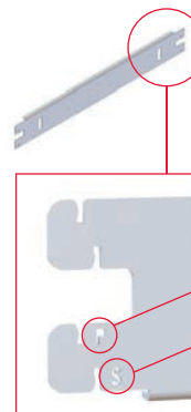
TIRANTES DISTANCIADORES. TIRANT-ESPACEMENT ROD-SPACER TIRANTE-DISTANZIATORE 4821/50B EJE 512 MM 4821/60B EJE 670 MM 4821/70B EJE 730 MM 4821/80B EJE 820 MM 4821/10B EJE 1000 MM
