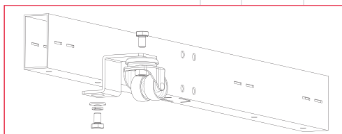
TIRANTES DISTANCIADORES TIRANT-ESPACEMENT ROD-SPACER TIRANTE-DISTANZIATORE 4821/50B eje 512 mm 4821/60B eje 670 mm 4821/70B eje 730 mm 4821/80B eje 820 mm 4821/10B eje 1000 mm
