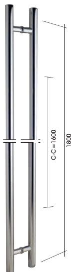
MANILLA DOBLE 180 CM POIGNÉE DOUBLE 180 CM DOUBLE DOOR HANDLE 180 CM MANIGLIA DOPPIA 180 CM 1591/02.
