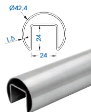
PERFILO PASAMANO Ø42.2 PROFIL GARDE-CORPS BALUSTRADE PROFIL PROFILO BALAUSTRRA INOX 316L *5100/122 Ø 42,4 mm
