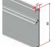
TAPA DE CARRIL SUPERIOR COUVERTURE DE RAIL SUPERIEURE TOP RAIL COVER COPERTURA SUPERIORE DEL BINARIO *3471/101 FACTURACIÓN EN 2M, 3M Y 4M.
