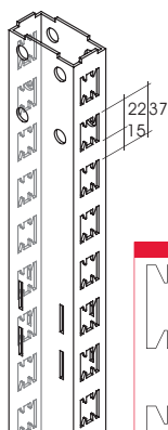
COLUMNA TROQUELADA 2 CARAS COLONNE PERFORATION SIMPLE 2 CÔTÉS UPRIGHT SINGLE SLOT CHANNEL 2 SIDES PIANTANA PERFORAZIONE SINGOLA 2 LATI 4815/26B 2678 mm
