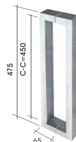
MANILLA DOBLE 47,5 CM POIGNÉE DOUBLE 47,5 CM DOUBLE DOOR HANDLE 47,5 CM MANIGLIA DOPPIA 47,5 CM 1596/028
