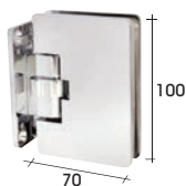
BISAGRA AUTOMÁTICA PARED-VIDRIO CHARNIERE AUTOMATIQUE MUR-VERRE AUTOMATIC HINGE WALL-GLASS CERNIERA AUTOMATICA PARETE-RETRO *4152/0.. latón
